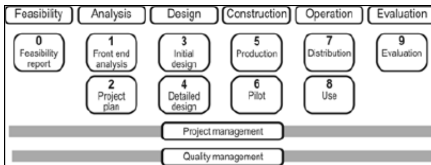
Figura 2: Metodología SSADM
