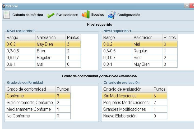
Figura 4 Interfaz de las escalas a utilizar en el cálculo de las métricas
